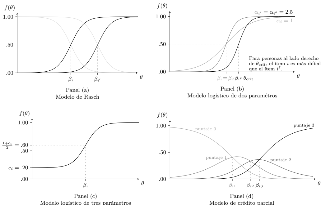
Figura 1. Curvas características en distintos modelos de respuesta al ítem
